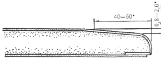
Рисунок 4 - Полукруглая и утоненная с лицевой стороны кромка (ШЛУК)
