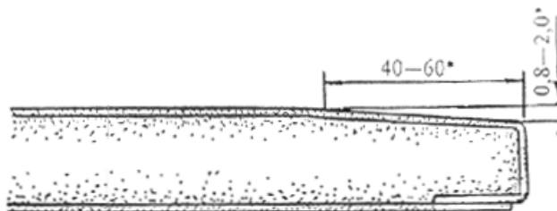
Рисунок 2 - Утонченная с лицевой стороны кромка (УК)
