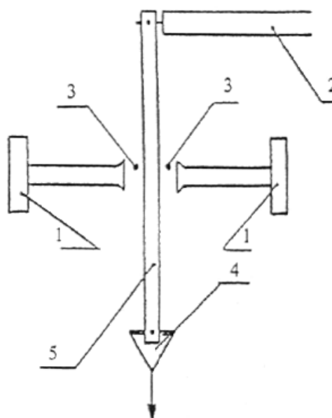
1 - горелка; 2 - рама; 3 - термопара; 4 - устройство для подвешивания груза; 5 - образец
